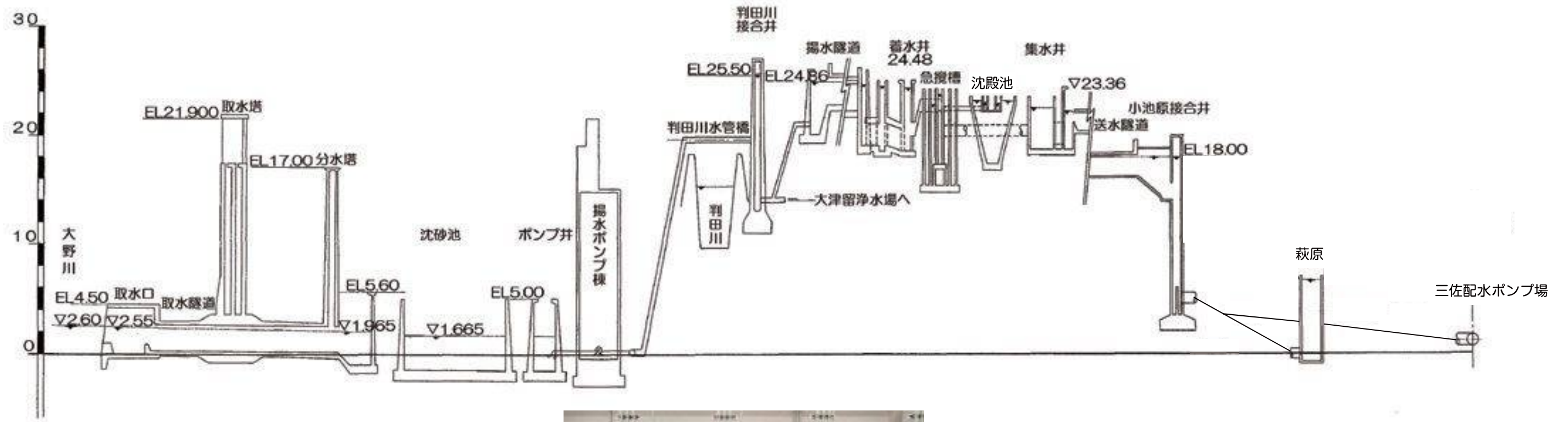
判田浄水場送水系統図
