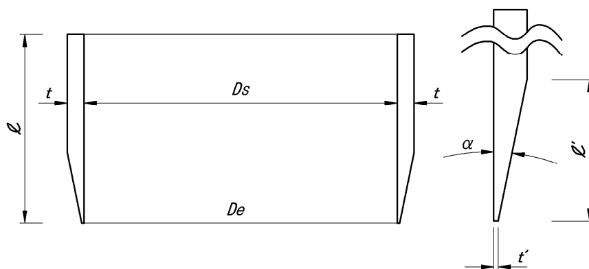
図2-1 サンプリングチューブ
