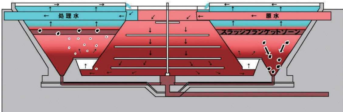
沈澱池断面図
