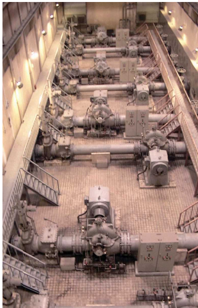
揚水ポンプ
