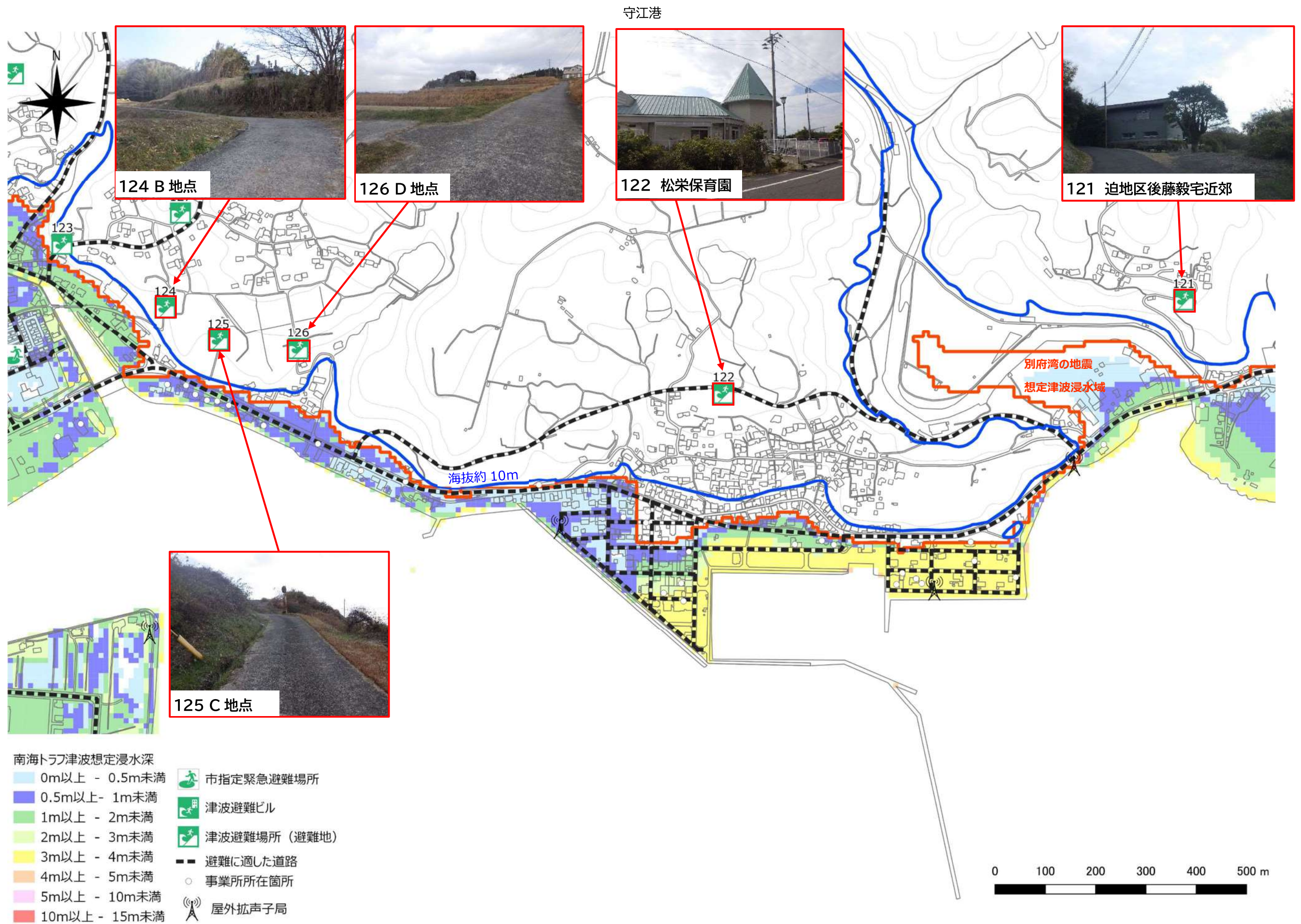
図 5-2 避難経路等と避難施設等の参考例 守江港 港湾津波避難計画 港湾地域【D】 P13
