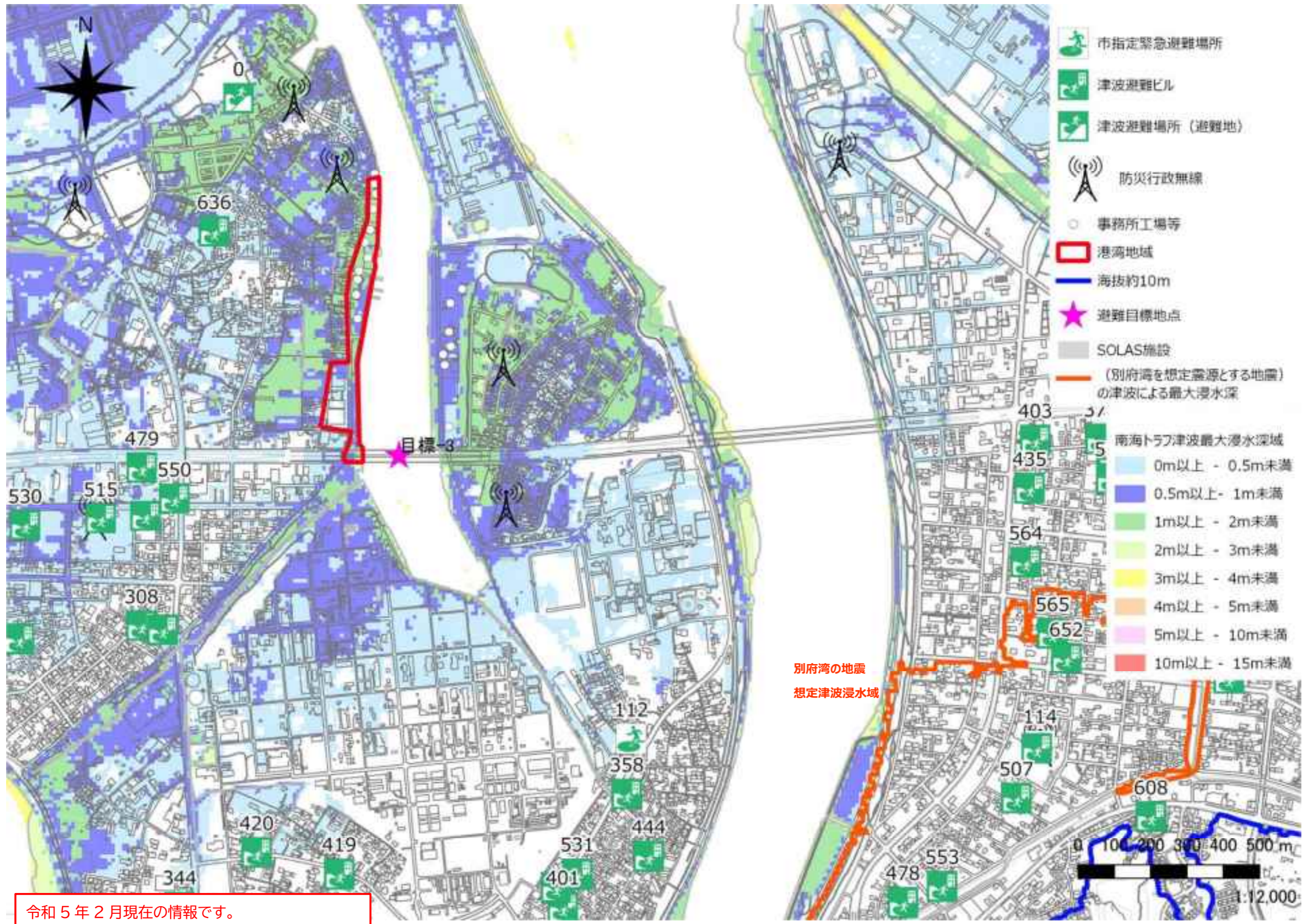
図4-1 港湾地域Iの詳細
