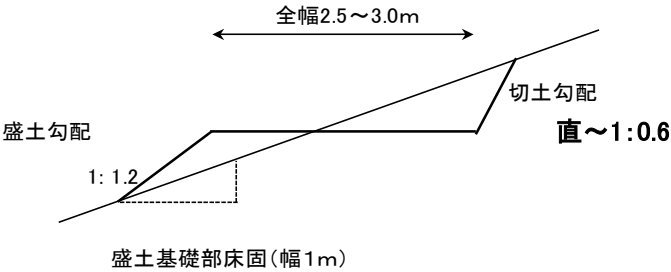
土工標準図
