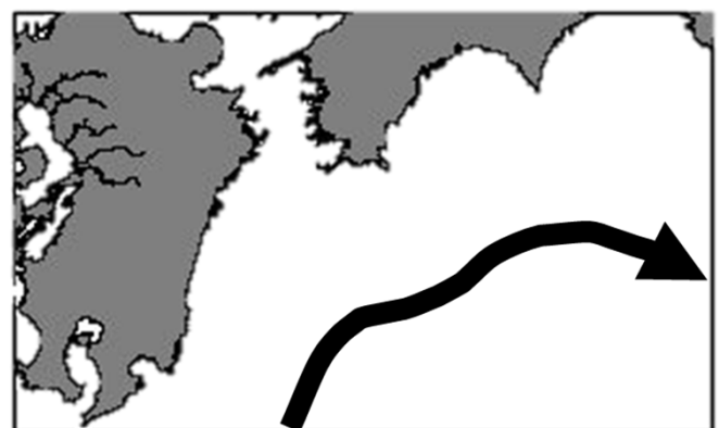
黒潮流路図
