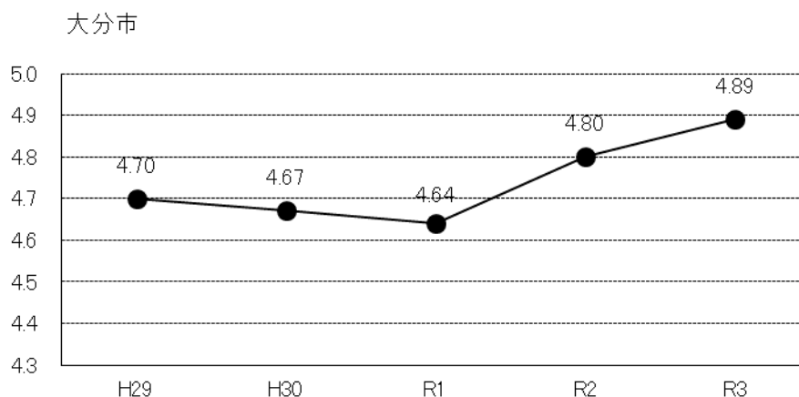
図7-1 雨水のpHの年平均値の経年変化
