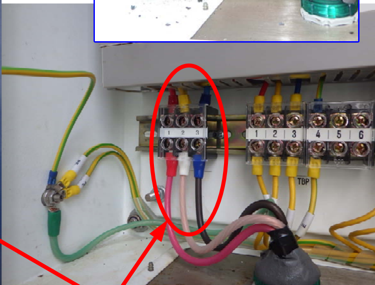
当該箇所 (変色したケーブルおよび端子台の取替実施)
