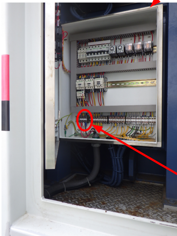
当該箇所 (変色したケーブルおよび端子台の取替実施)
