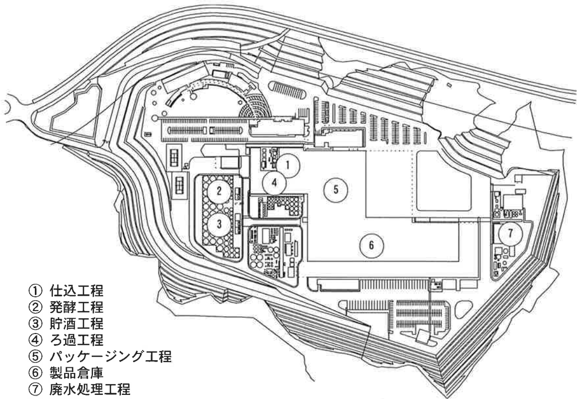
図3 工場配置図
