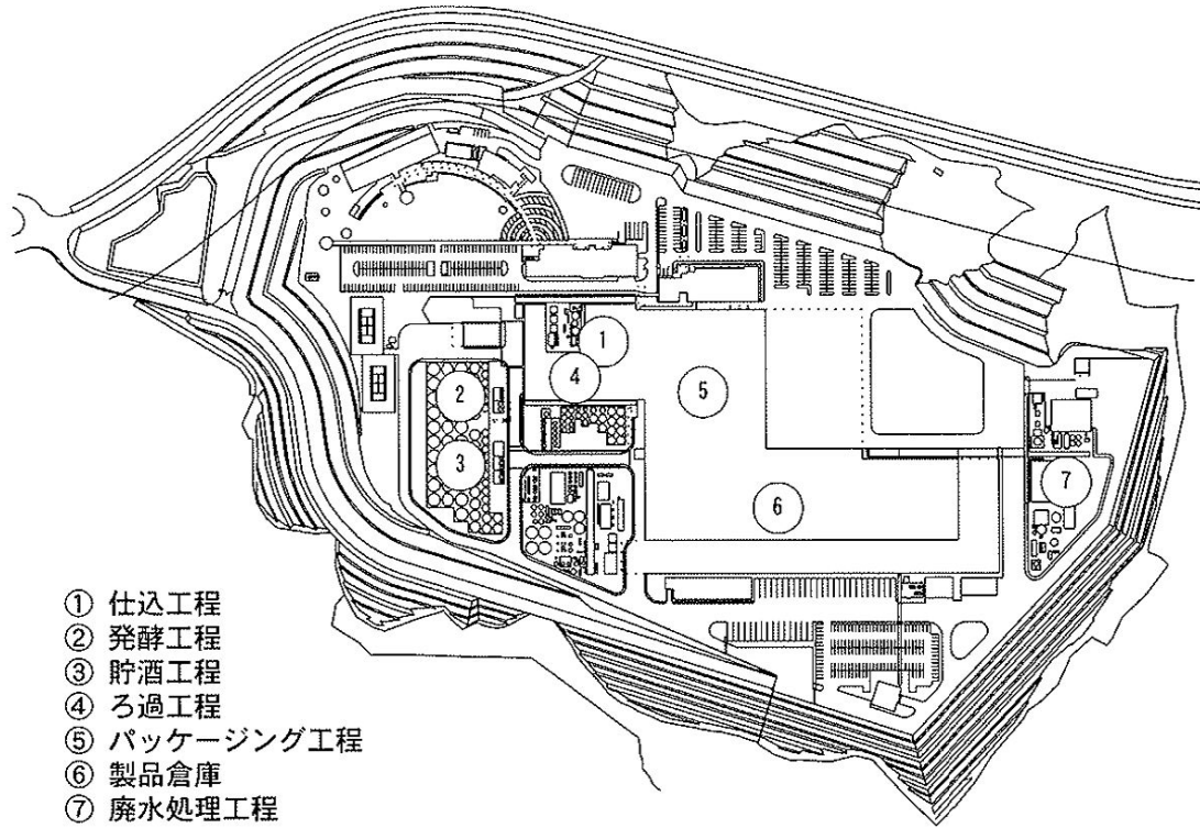
図3 工場配置図
